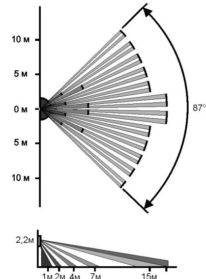
Рис.4 Диаграмма зоны обнаружения при наклоне основания извещателя вперед на 12 градусов
