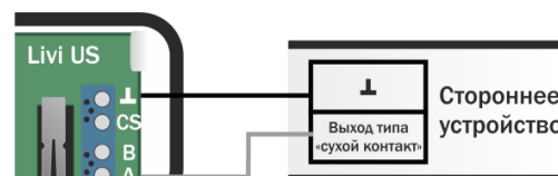
Рисунок 6.3 – Схема подключения одного устройства к датчику
