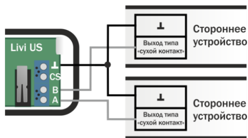
Рисунок 6.2 – Схема подключения двух устройств к датчику
