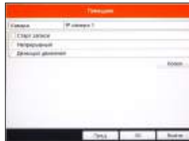
Рисунок 4.8 Настройка записи.
