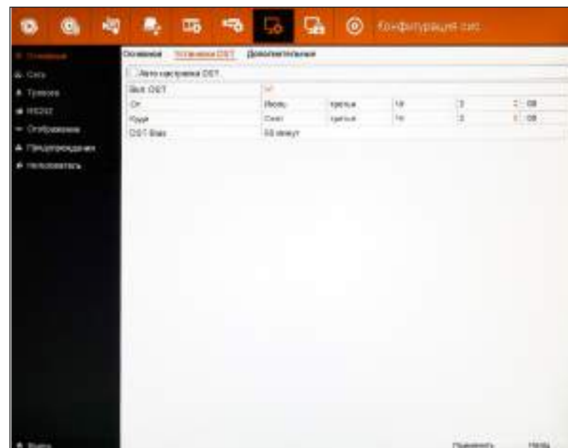
Рисунок 5.67 Установки DST.
