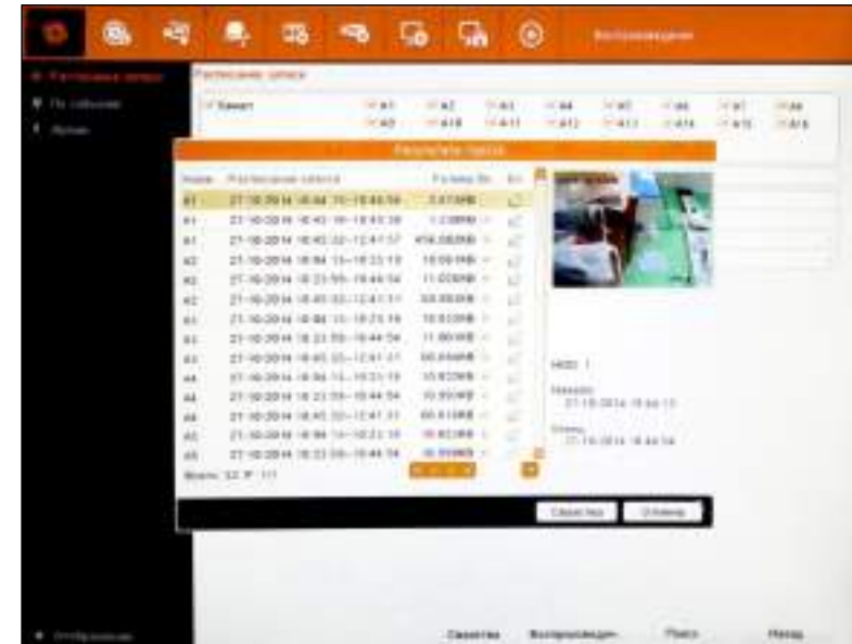
Рисунок 5.3 Найденные файлы.
