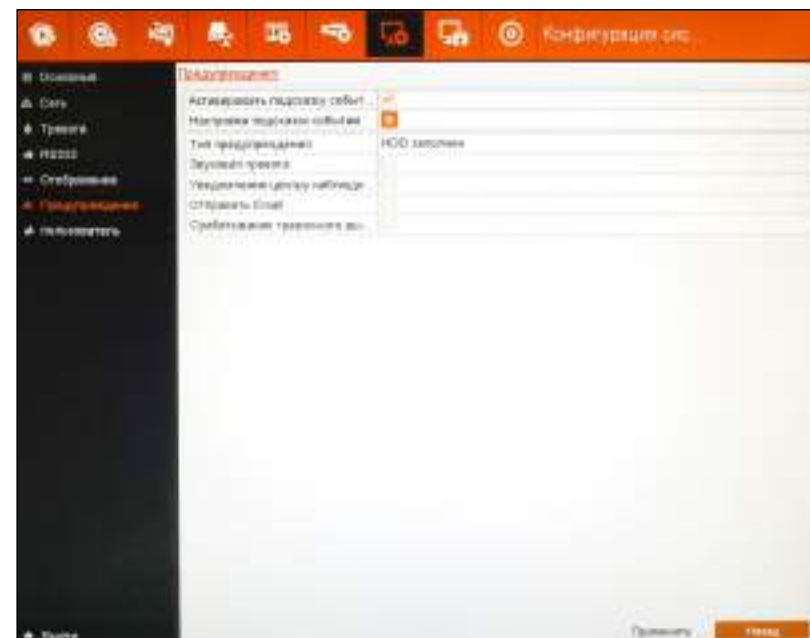
Рисунок 5.91 Предупреждения.
