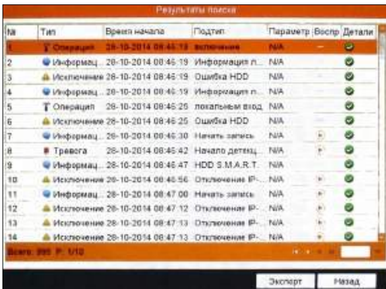
Рисунок 5.102 Список событий.
