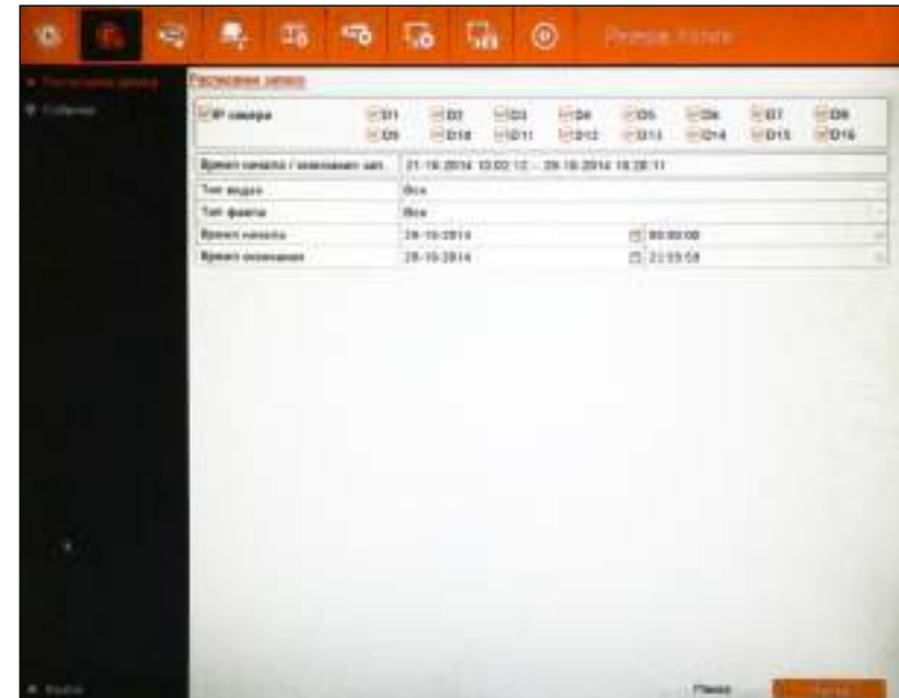
Рисунок 5.1 Расписание записи.
