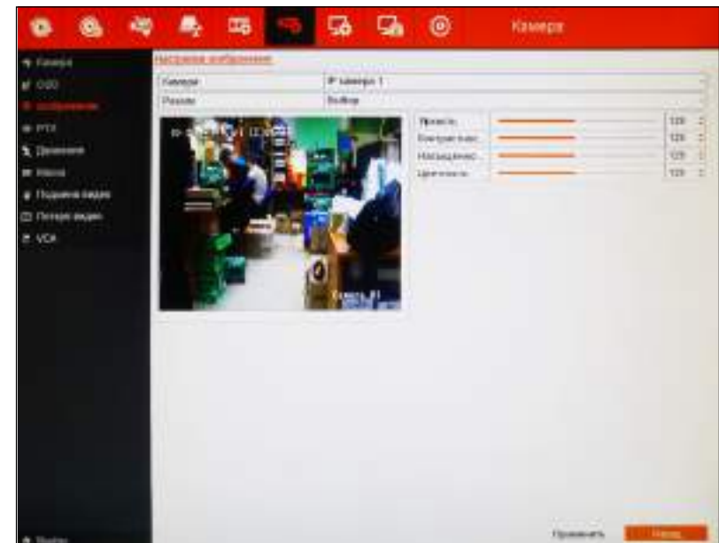
Рисунок 5.50 Настройка изображения.
