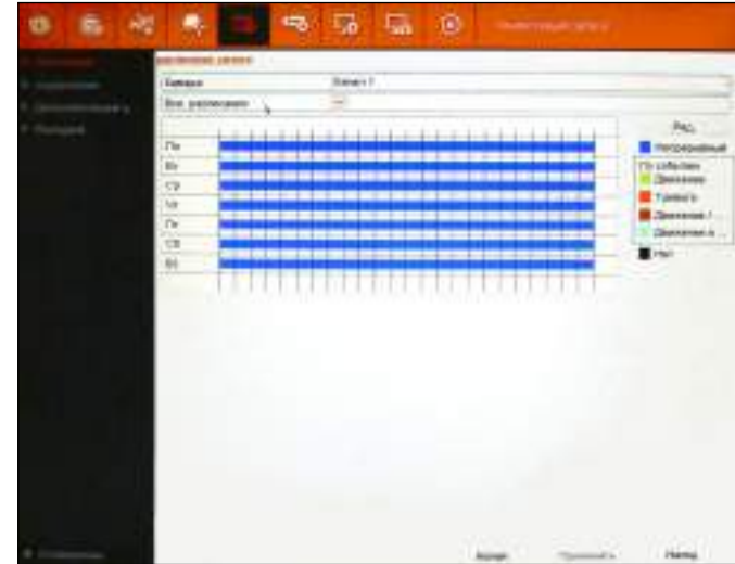
Рисунок 5.32 Расписание.
