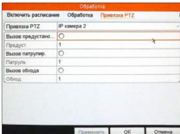
Рисунок 5.83 Привязка PTZ.
