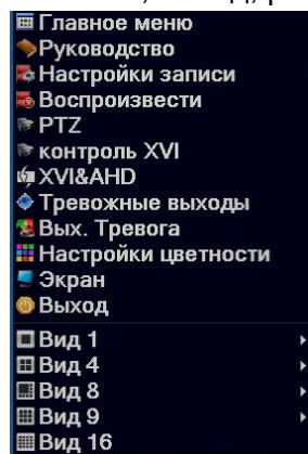
Рис 3.2 Контекстное меню
