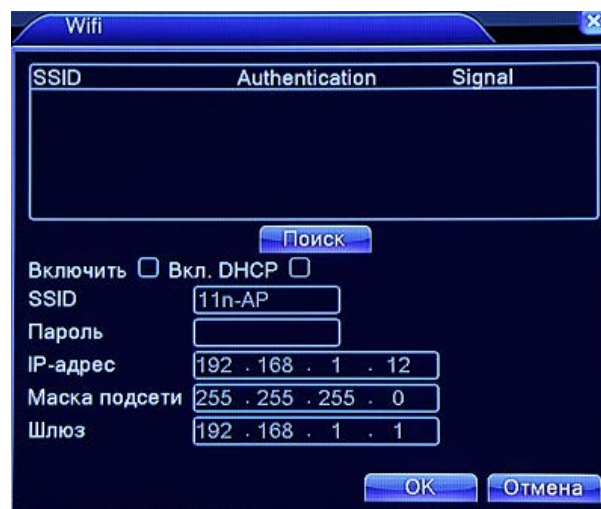
Рис. 4.34 Настройка Wi-Fi
