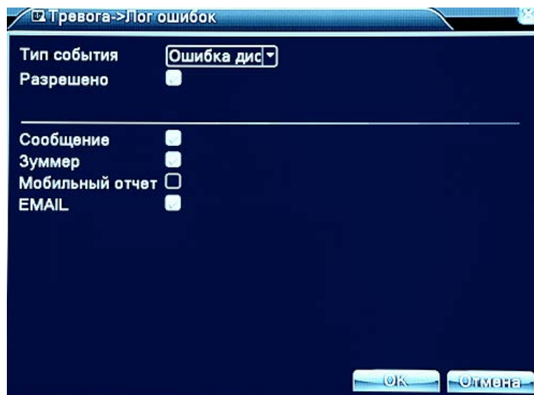
Рис 4.11 Диагностика неисправностей
