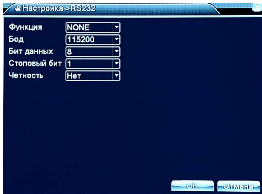
Рис. 4.39 Настройка RS232
