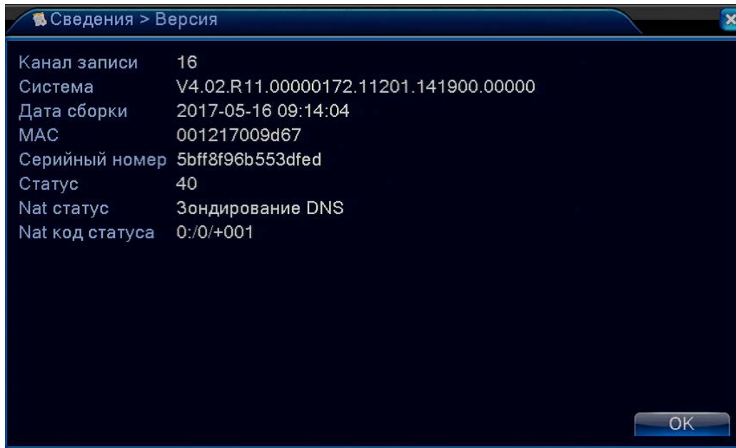
Рис 4.56 Версия ПО
