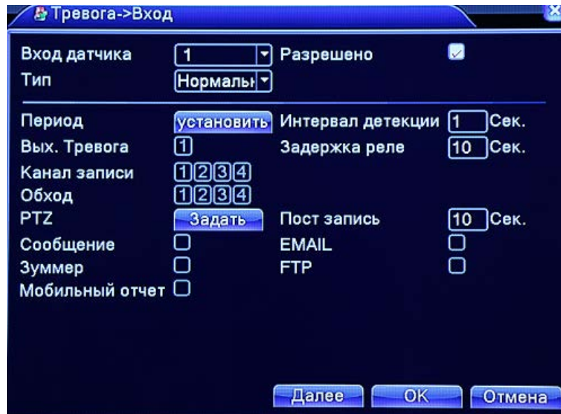
Рис. 4.10 Сигнал тревоги
