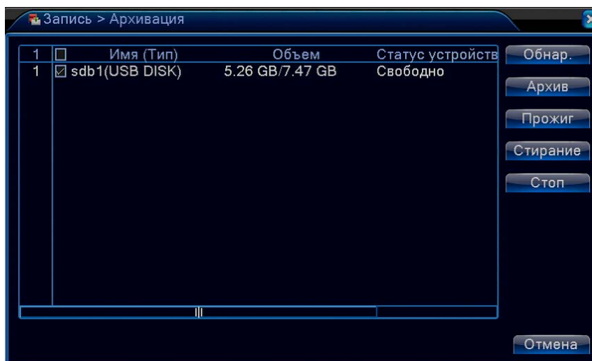
Рис. 4.3. Копирование
