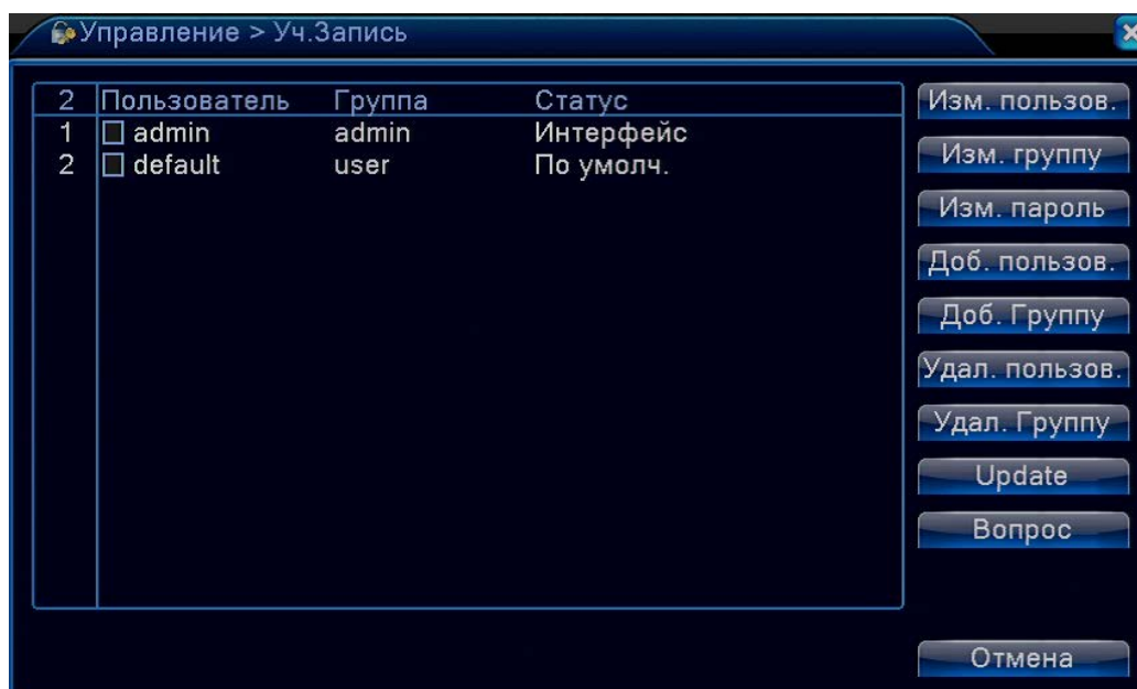
Рис. 4.42 Учетные записи
