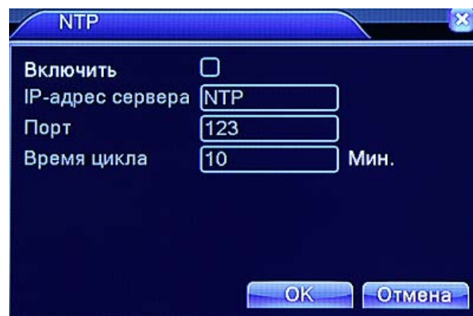
Рис. 4.25 NTP сервер
