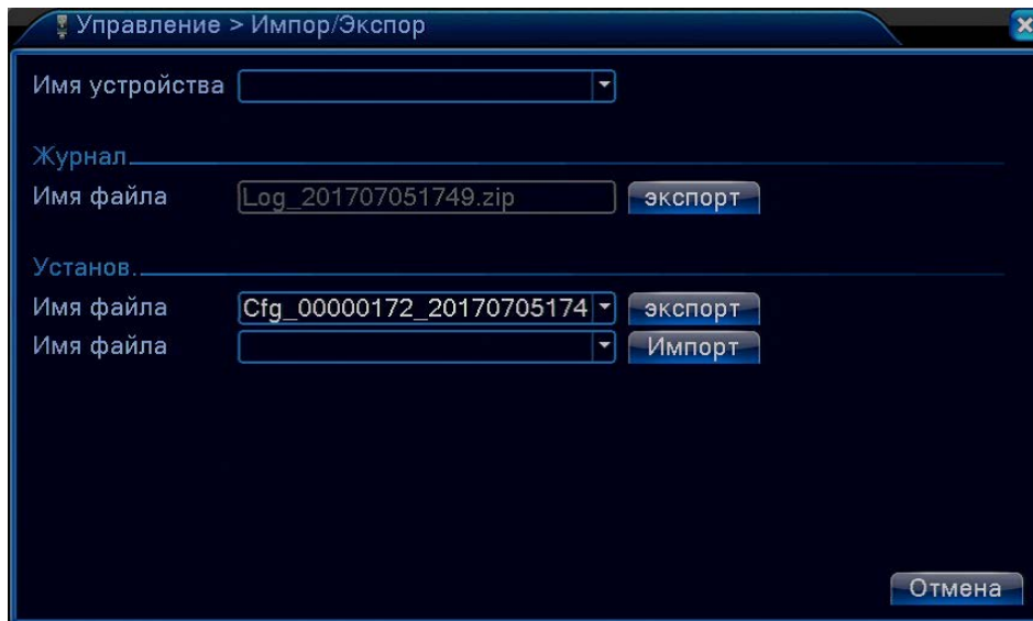
Рис 4.53 Импорт/экспорт
