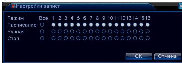
Рис 3.8 Режим записи
