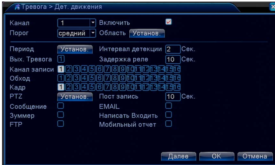
Рис 4.4 Обнаружение движения
