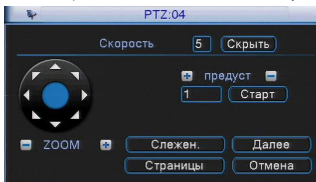
Рис. 3.10 Управление PTZ
