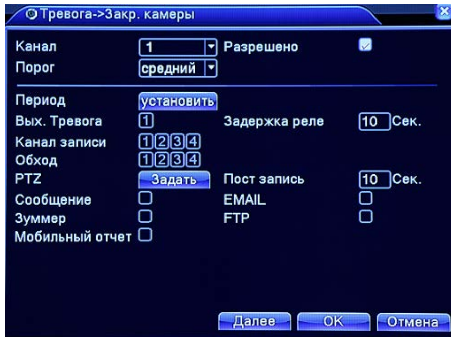
Рис 4.8 Закрытие камеры
