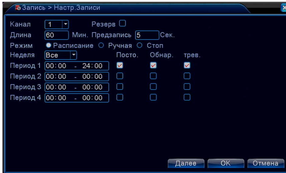
Рис 4.1 Настройка записи
