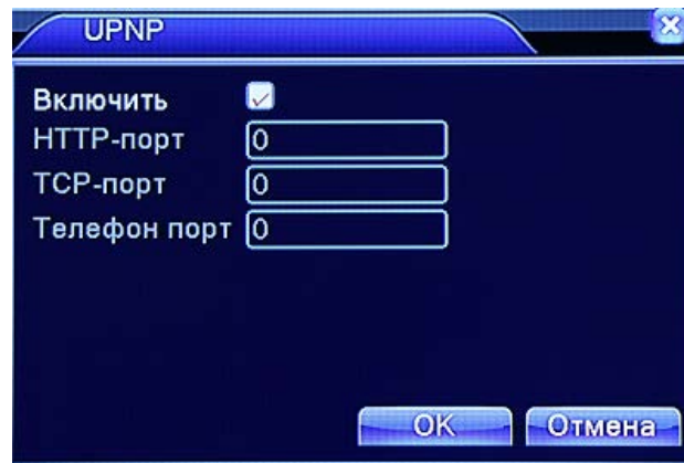
Рис. 4.33 UPNP
