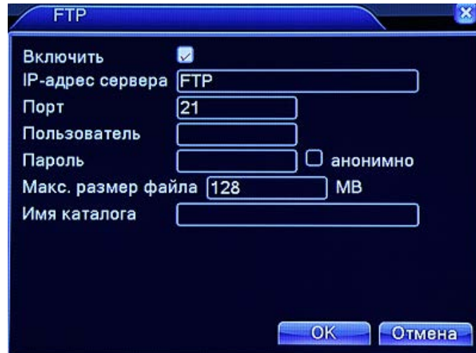
Рис. 4.29 Настройки FTP
