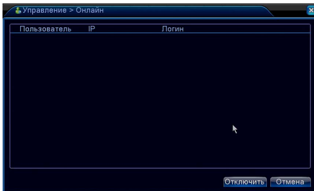
Рис 4.48 Online-пользователи
