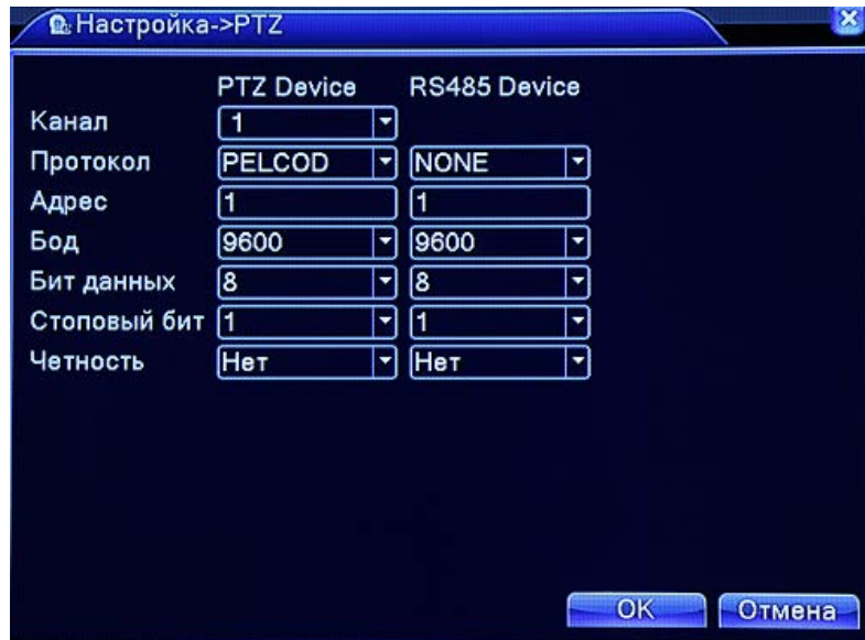
Рис. 4.38 Настройка PTZ
