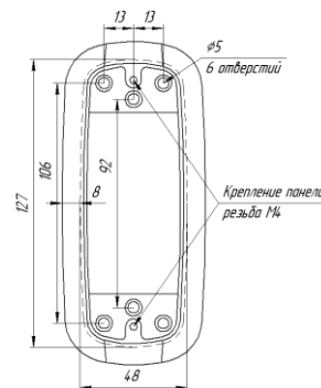
Установочные размеры врезного кронштейна
