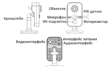
Рисунок 1-26 Компактная камера
