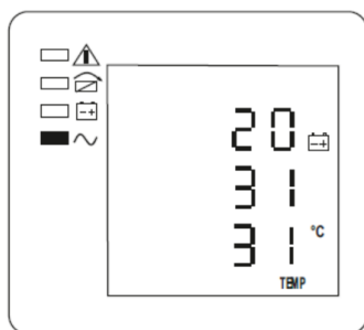
Рисунок 18 — ЖК-дисплей, температура АКБ, внутренняя и внешняя температура
