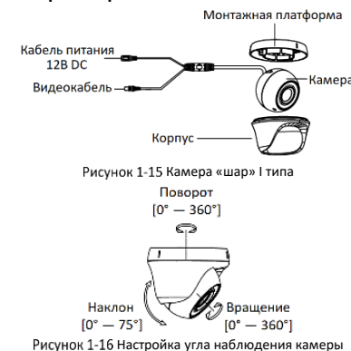
Рисунок 1-16 Настройка угла наблюдения камеры
