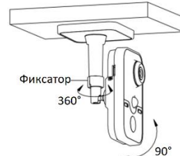
Рисунок 1-27 Настройка угла наблюдения камеры
