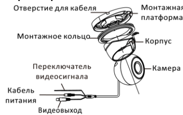
Рисунок 1-20 Камера «шар» V типа
