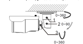
Рисунок 1-8 Настройка угла наблюдения камеры
