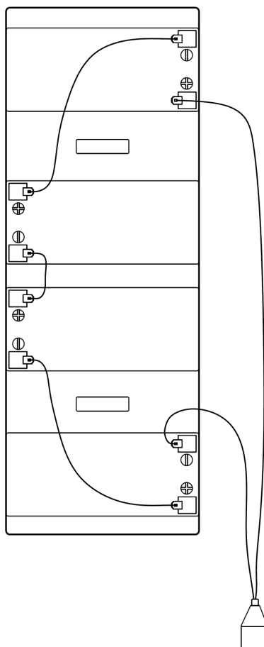
Рисунок 7 — схема соединений АКБ
