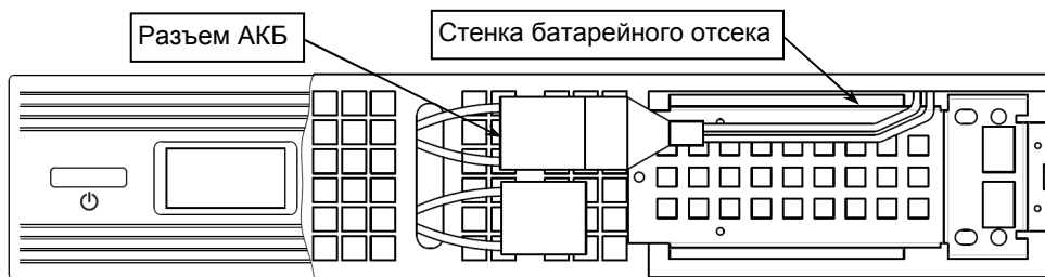
Рисунок 5 – Подключение внутренних батарей
