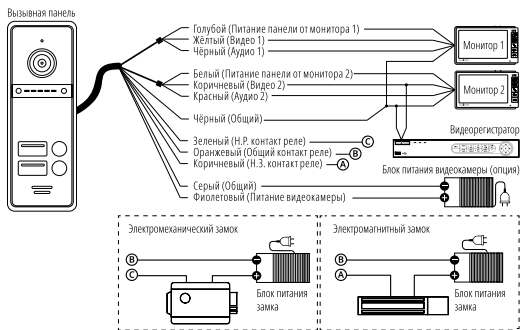
Рис. 16 Схема подключения вызывной панели FANTASY 2 HD
