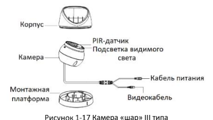
Рисунок 1-17 Камера «шар» III типа
