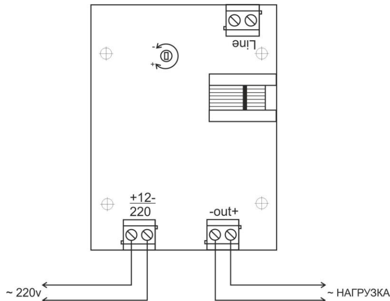
Рисунок 2. Внешний вид платы приставки дублирования сигнала вызова GC-0001D2
