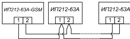
Рисунок 3 – Схема соединения извещателей в группу
