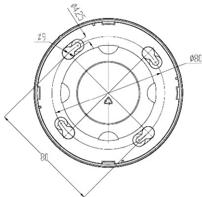
Рисунок 1 – Расположение отверстий для крепления базы извещателя
