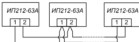
Рисунок 2 – Схема соединения извещателей в группу
