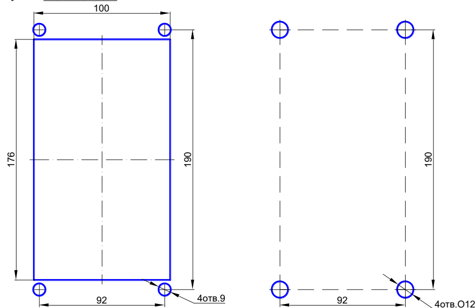
Рис1. Разметка под крепление DP7000ip-Hybrid/IPC VBS а) снаружи; б) изнутри.
