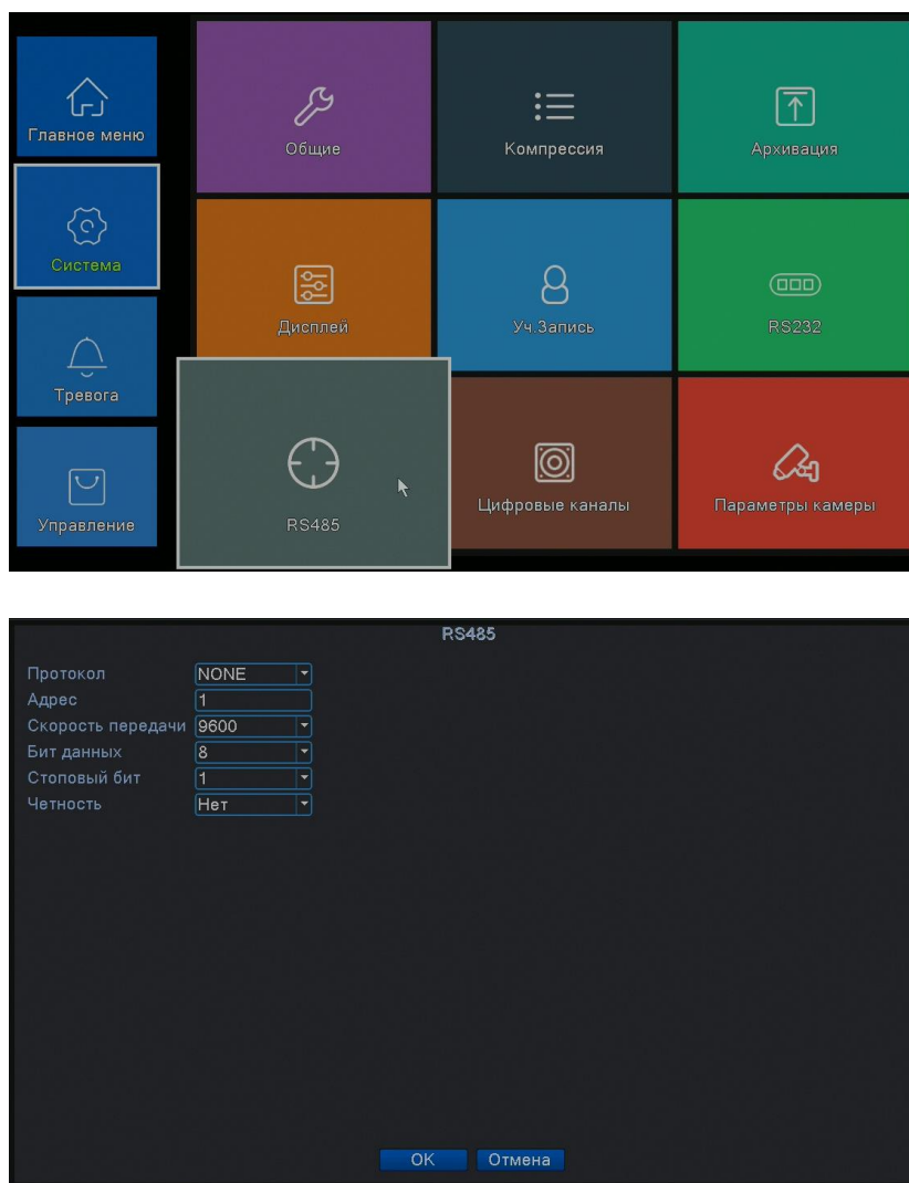
Рисунок 4.37 Конфигурация RS485 устройств в цифровом режиме.
