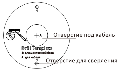
Рисунок 2-2 Шаблон крепления
