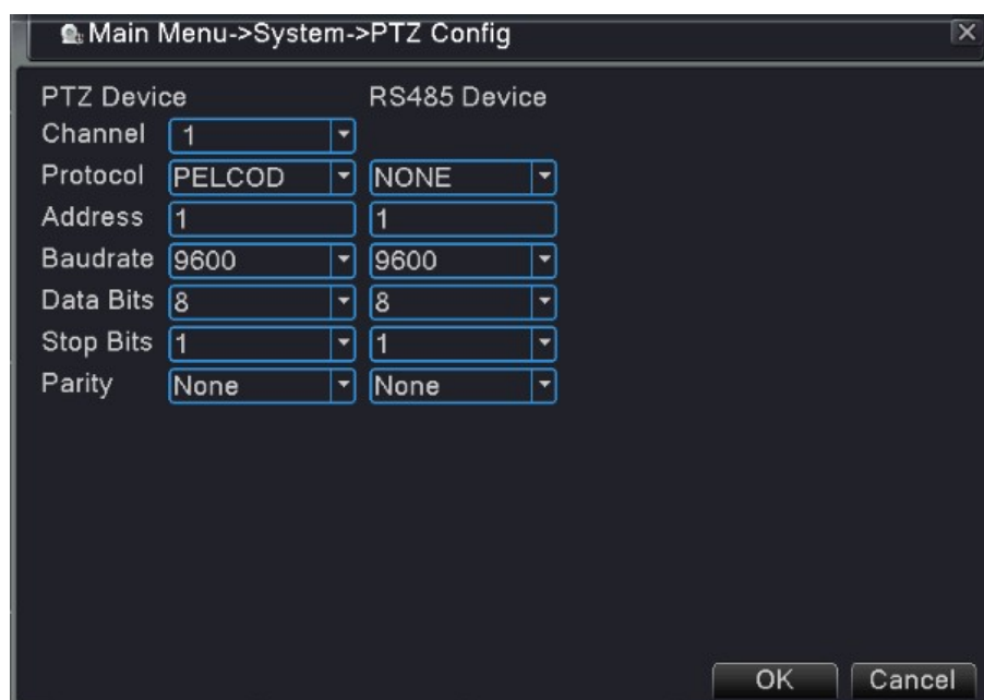
Рис. 4.31 Конфигурация PTZ
