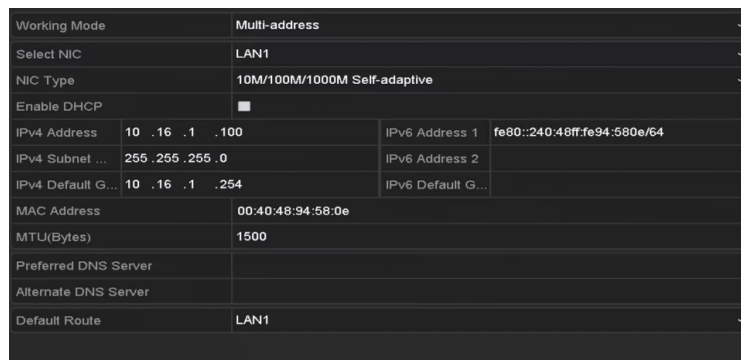
Рисунок 3.12 Сетевые параметры
