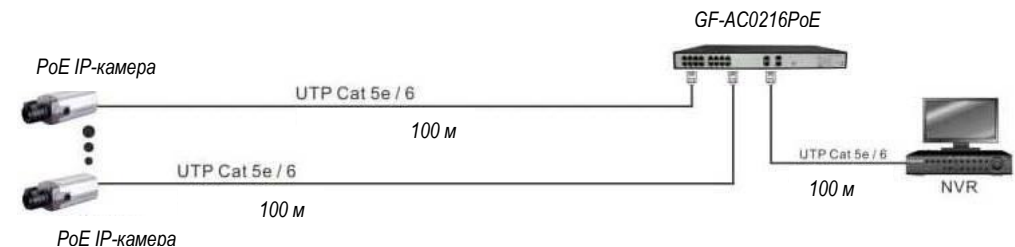
Рис. 1 Схема подключения сетевых устройств
