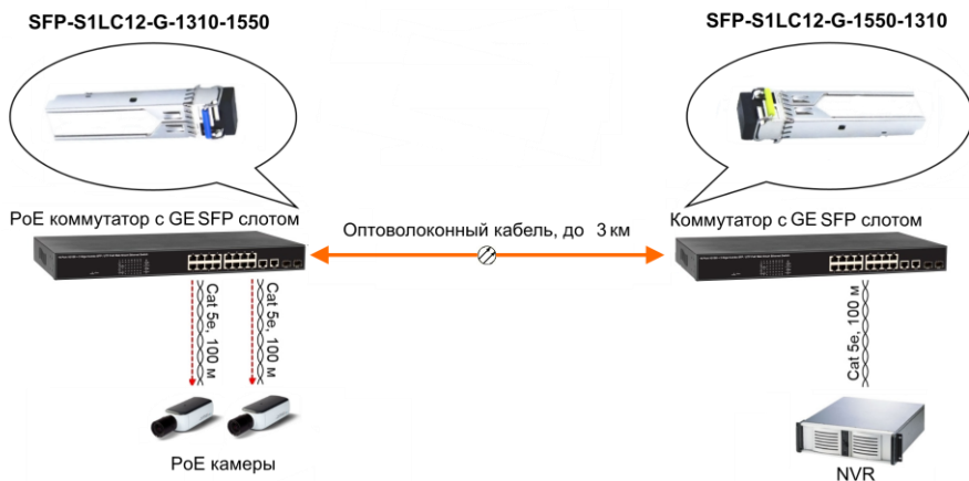
Рис.4 Типовая схема подключения SFP модулей SFP-S1LC12-G-1310-1550, SFP-S1LC12-G-1550-1310
