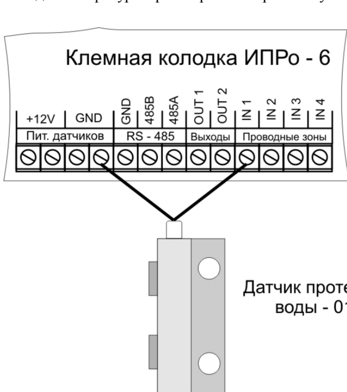
Подключение 1 датчика
