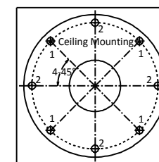
Рисунок 2-1 Шаблон крепления
