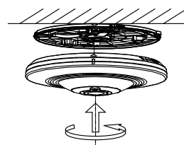
Рисунок 1-29 Настройка угла наблюдения камеры
