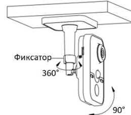
Рисунок 1-27 Настройка угла наблюдения камеры
