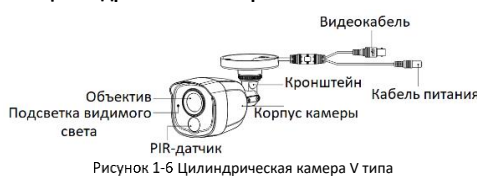
Рисунок 1-6 Цилиндрическая камера V типа
