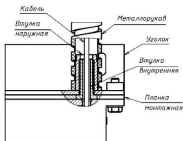
Рисунок 4 – Устройство кабельного ввода
