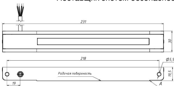
Рисунок 2 - Корпус
