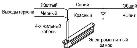
Рисунок 6 – Схема подключения замка
