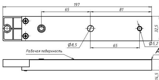
Рисунок 3 - Якорь
